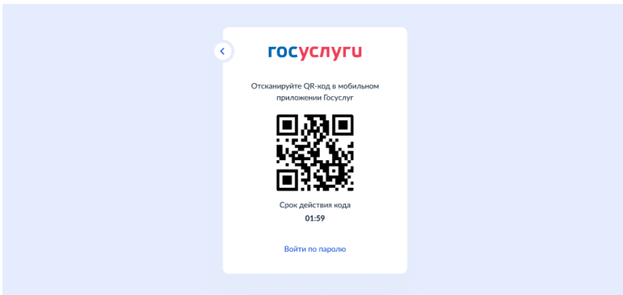
Рисунок 98 – Отображение QR-кода
