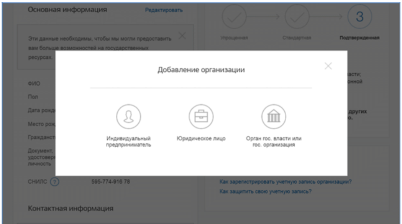
Рисунок 59 – Добавление организации
