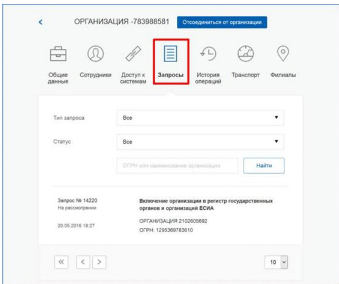
Рисунок 136 – Перечень запросов
