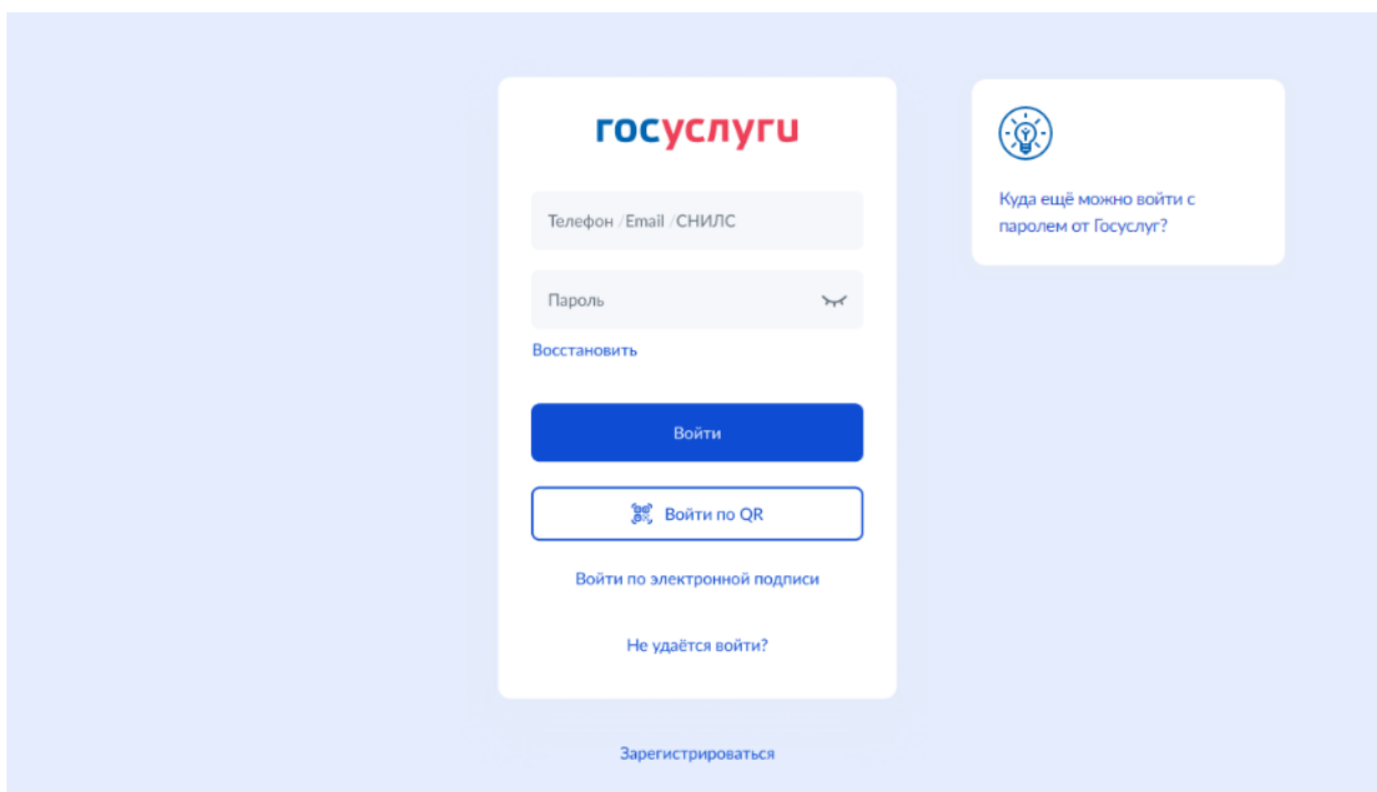
Рисунок 88 – Страница авторизации
